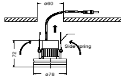
Deckeneinbauleuchte
